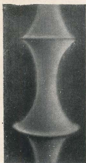
Псевдосферические поверхности, на которых осуществляется геометрия Лобачевского.
